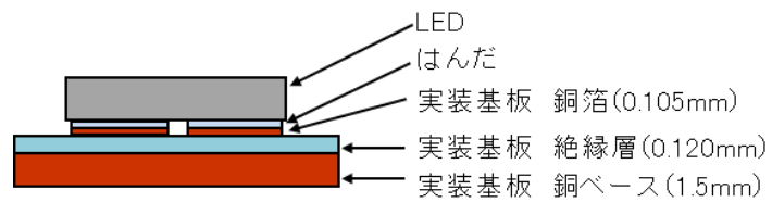
図3 実装構造
